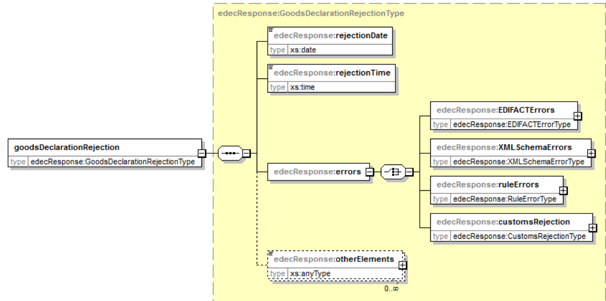
Abbildung 33: goodsDeclarationRejection mit Child Elements
