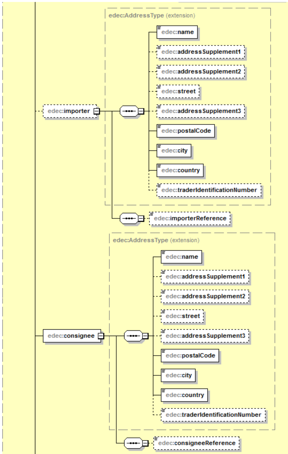
Abbildung 19: goodsDeclaration mit aufgeklappten Child Elements (Teil 5)
