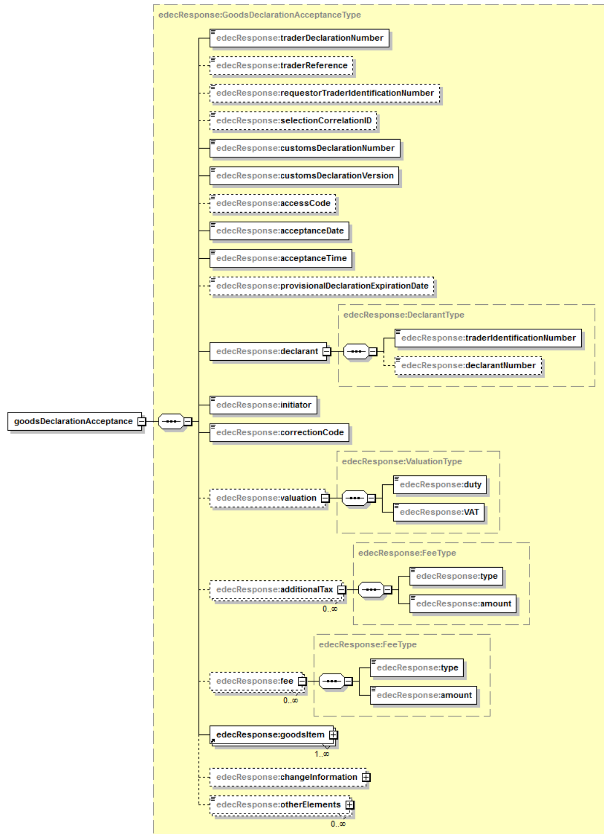
Abbildung 31: goodsDeclarationAcceptance mit aufgeklappten Child Elements
