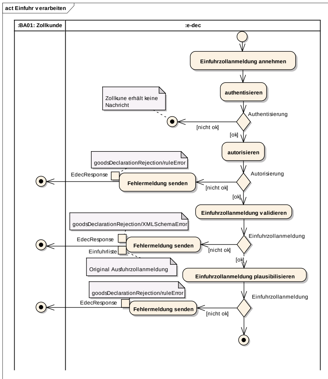
Abbildung 2: Einfuhrzollanmeldung verarbeiten
