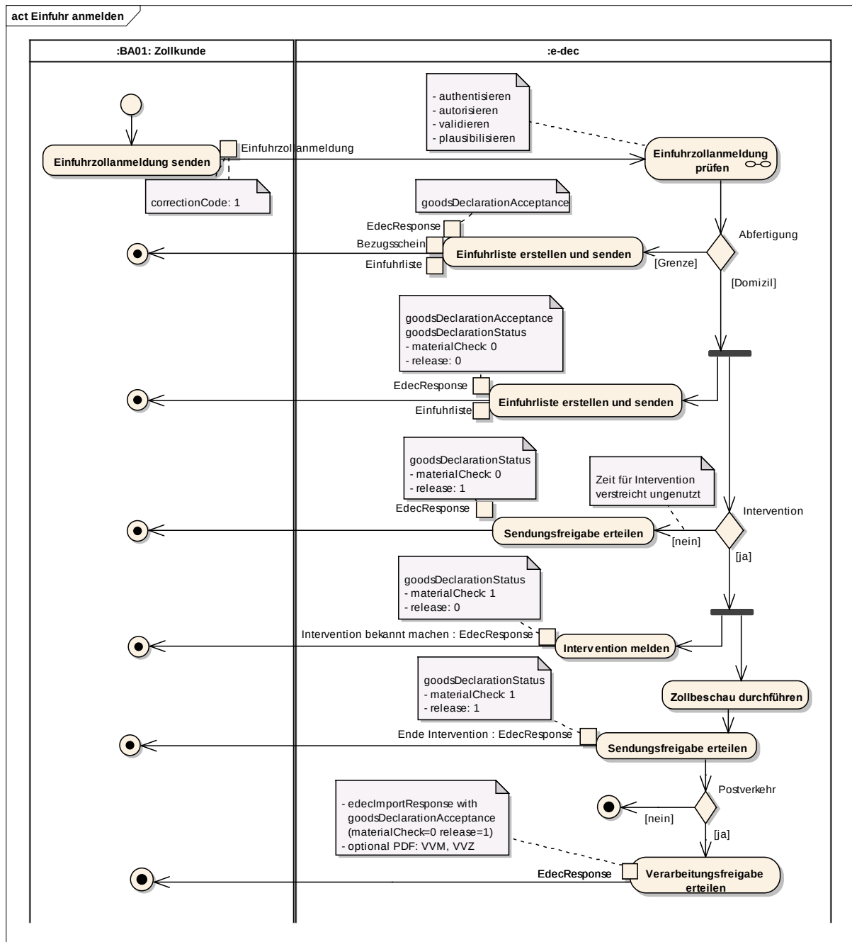
Abbildung 1: Aktivitätsdiagramm für Einfuhrzollanmeldung übermitteln
