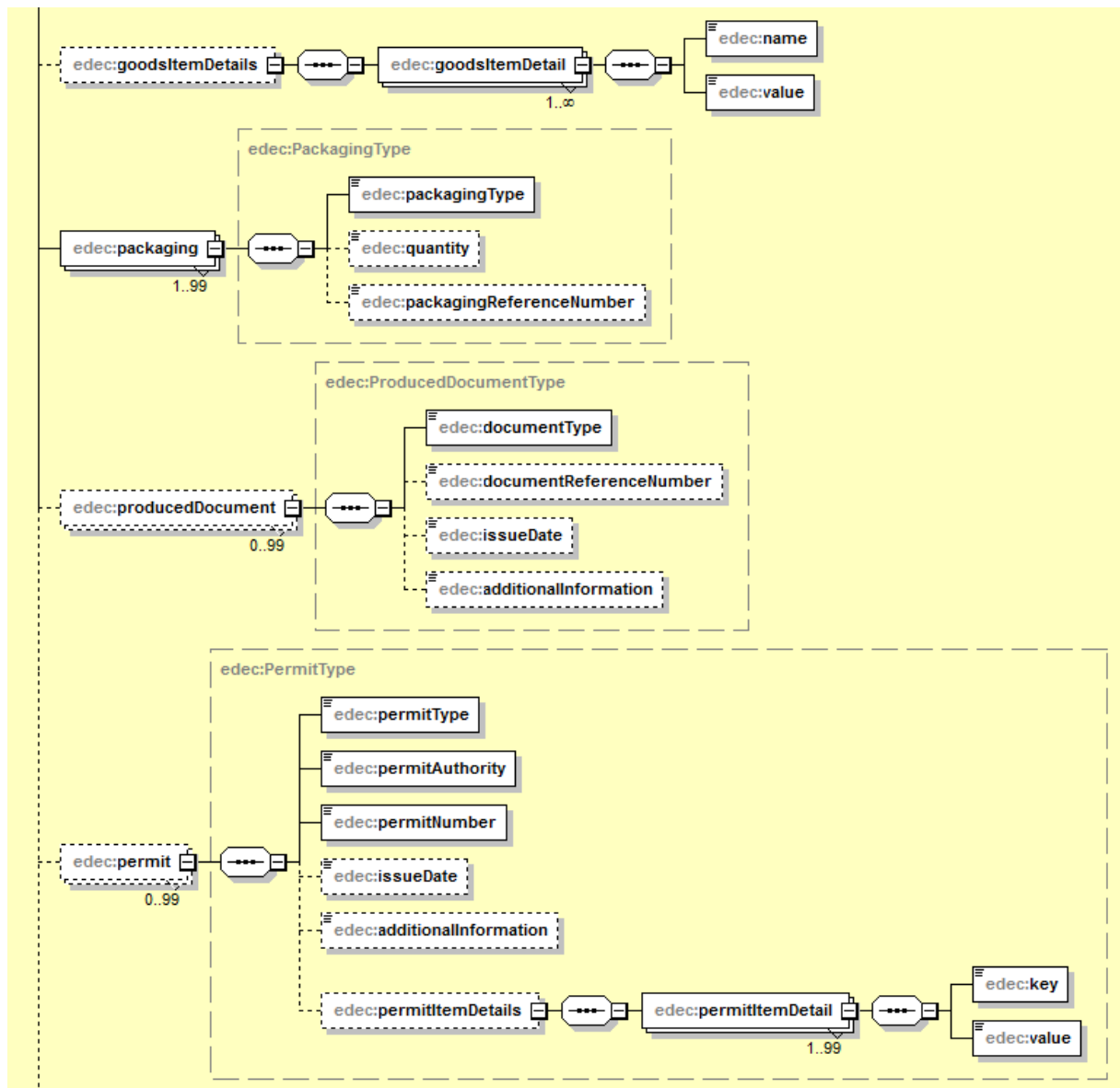
Abbildung 26: goodsItem mit aufgeklappten Child Elements (Teil 3)
