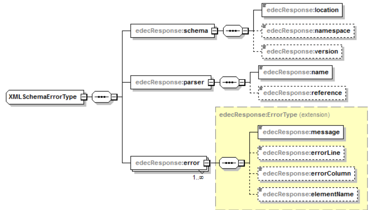
Abbildung 34: XMLSchemaError mit aufgeklappten Child Elements
