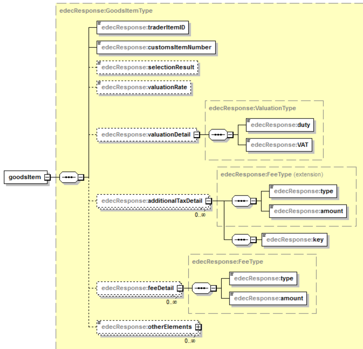
Abbildung 32: edecResponse GoodsItemType
