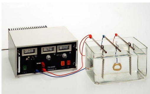
Petite installation de bijoutier pour les revêtements galvaniques sur bijoux. PHOTO : UBOS
