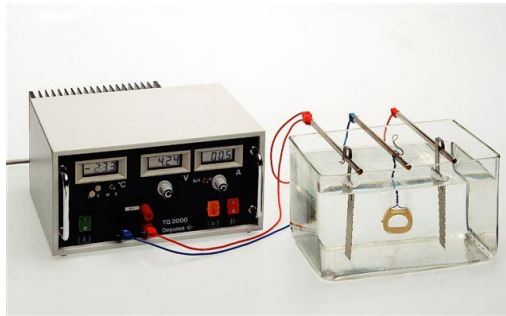
Kleinanlage für Goldschmiede für den galvanischen Überzug von Schmuck. BILD: UBOS
